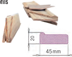
Profils
